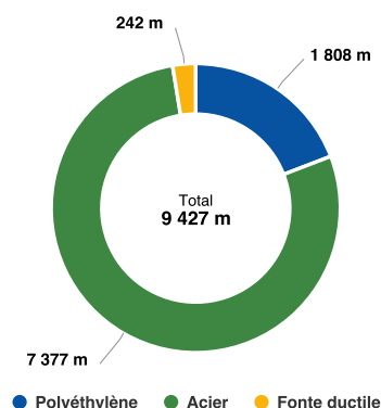
Canalisations par matière en 2021
